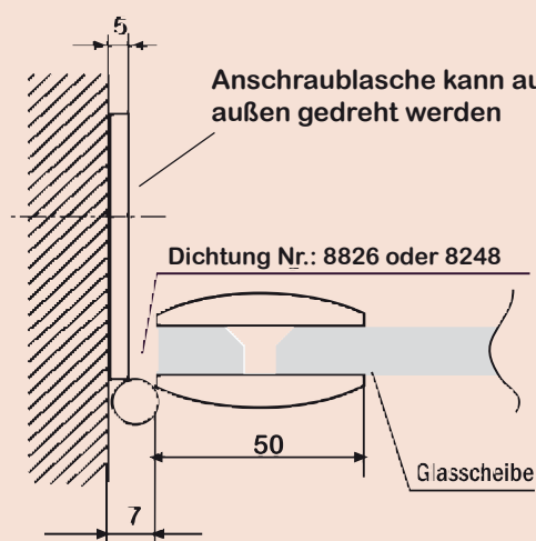
Anschraublasche außen
